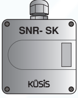
Karbondioksit Sensörü 0-10.000 ppm \pm 10 ppm
